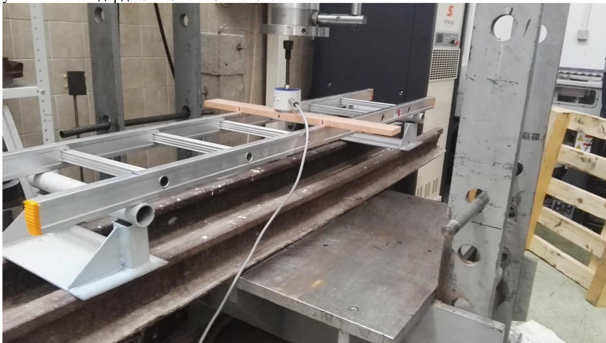
Слика 2 Конфигурација мерења носивости мердевина
