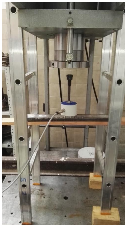
Слика 4. Фотографија са мерења оптерећењем на средини газишта
